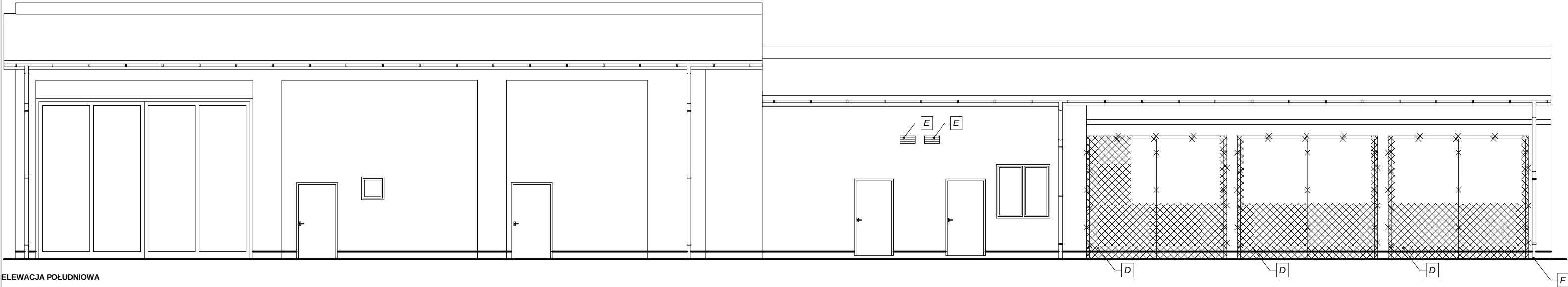
ELEWACJA POŁUDNIOWA
